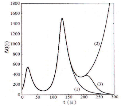
図2 新規陽性者数の予測。極端な状況がわかるようにパラメータを設定したもの。(1) 現在の接触制限を保った場合、(2) 制限緩和だけを行った場合。(3) 制限緩和に加えて、隔離を充実した場合。
