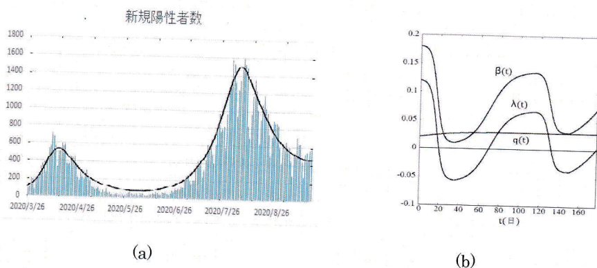
図 1 (a) 全国の新規陽性者数の日ごと変化。実線は、(4) 式によるフィッティング。データは厚生労働省による[14]。(b) フィッティングに用いた \beta(t) , q(t) および増減率 \lambda(t) の変化。 \gamma = 0.04
